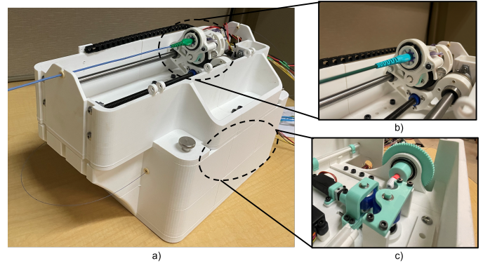
Fig. 1: 4 DoF Catheter Intervention Robot: Guide Catheter Module & Guidewire Module
